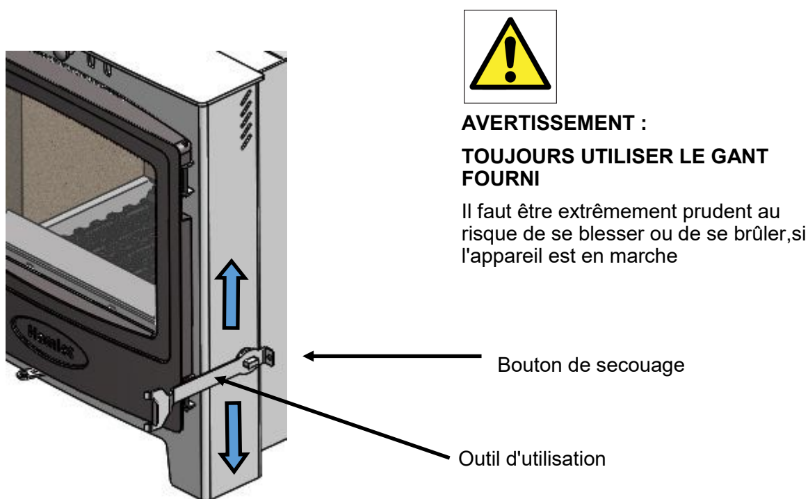
Fig. 6. Secouage de la grille
